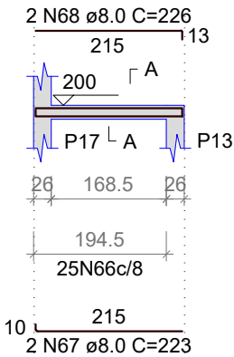
SEÇÃO A-A ESC 1:50
