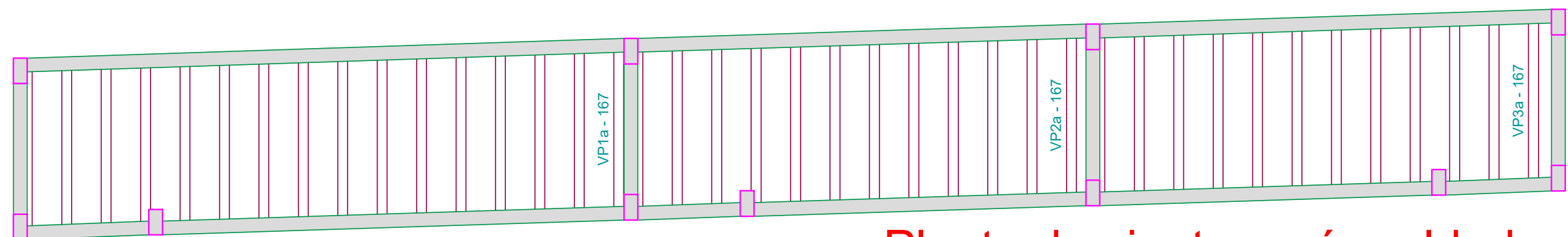
Planta de vigotas pré-moldadas escala 1:50
