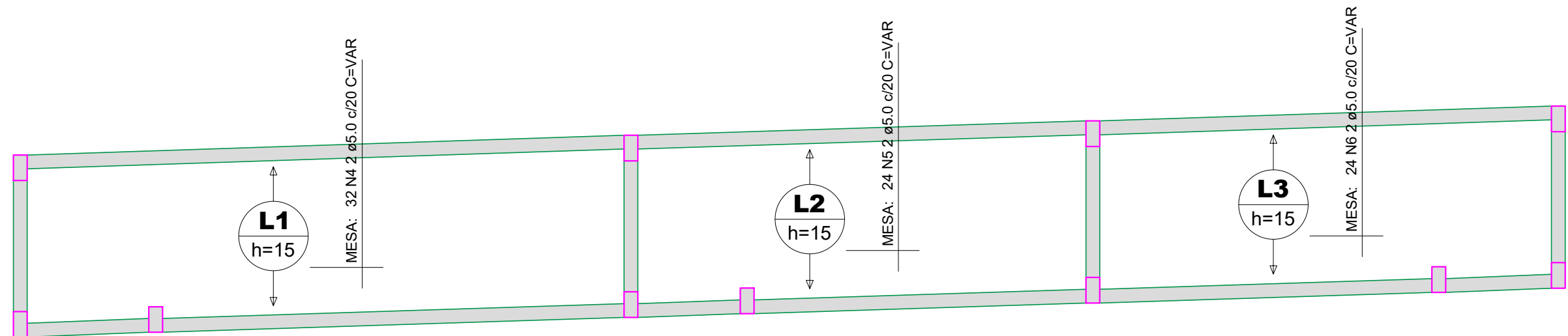
Armação positiva das lajes do pavimento Topo (Eixo Y) escala 1:50
