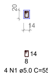
SEÇÃO A-A ESC 1:50
