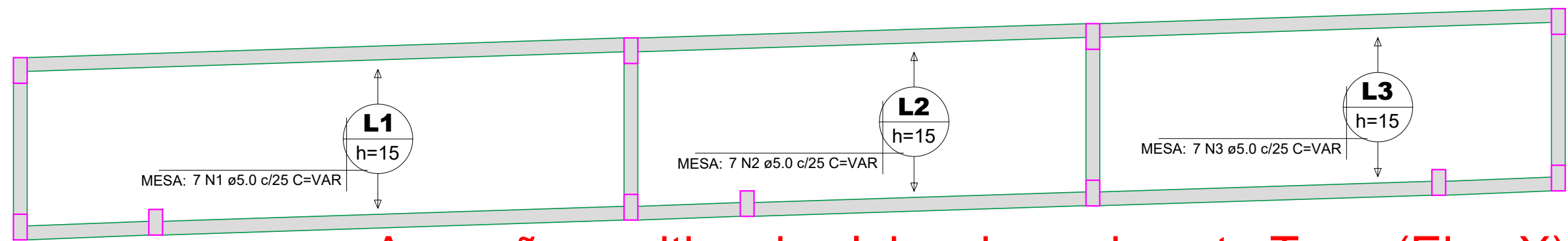
Armação positiva das lajes do pavimento Topo (Eixo X) escala 1:50
