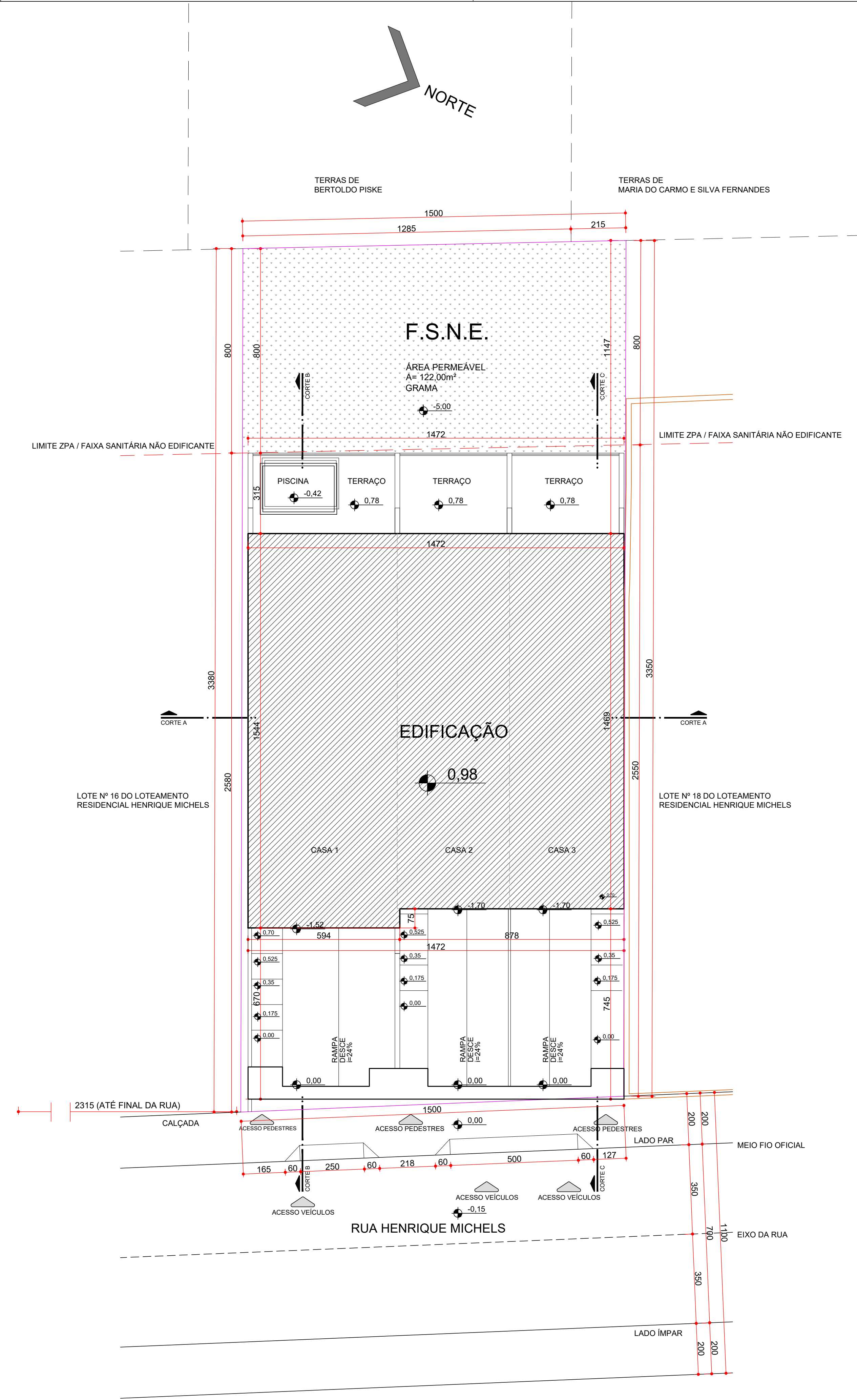
PLANTA DE SITUAÇÃO ÁREA TOTAL: 677,69m² ESCALA: 1/100
