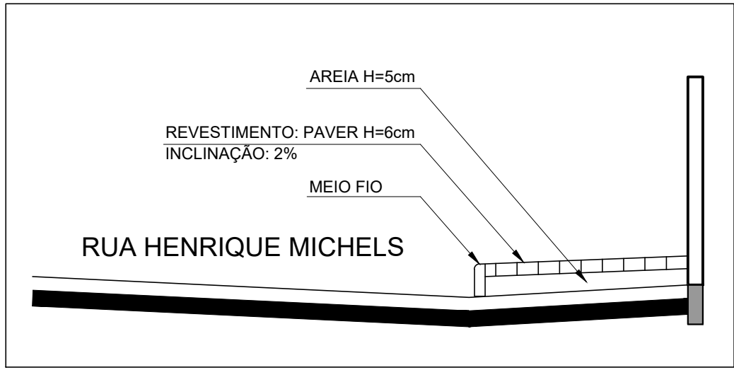
DETALHE CALÇADA ESCALA: 1/50
